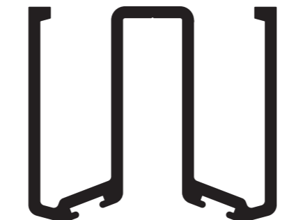
SD562 JAMB TRIM
